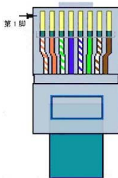
图 6 网线线序
