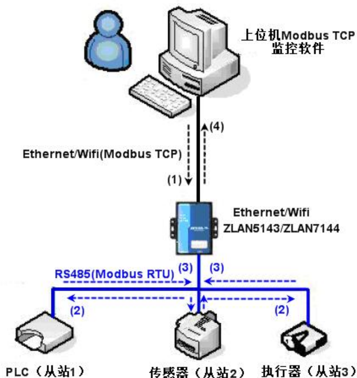
图 39 存储型 Modbus 网关工作方式
