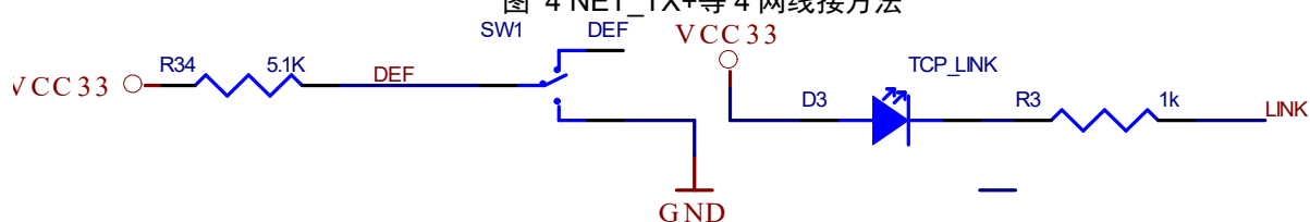
图 5 复位脚和 LED 引出方法
