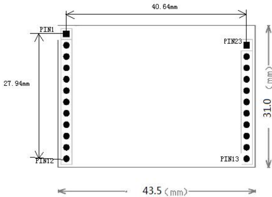
图 3 ZLSN7004 排针接口
