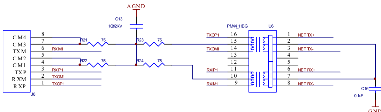
图 4 NET_TX+等 4 网线接方法
